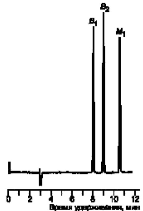
Рисунок 2 — Хроматограмма рабочего раствора смеси афлатоксинов
