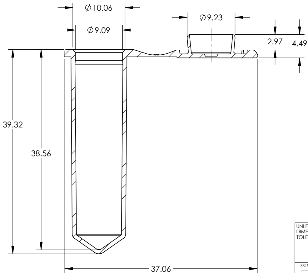
SECTION A-A SCALE: 2.2 : 1
