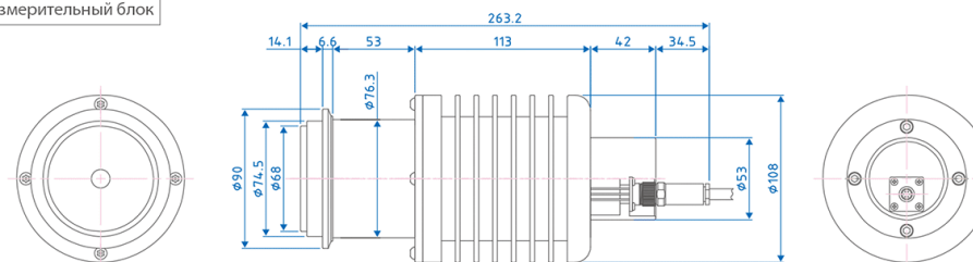
Измерительный блок
